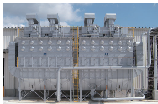
BFR4×6(37kW×2) 2基
